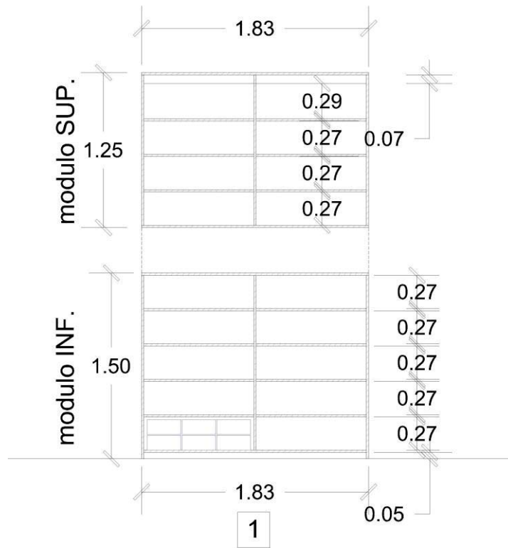
despiece modulo 1
