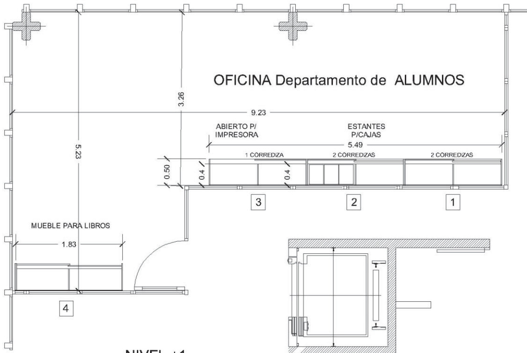
NIVEL +1 Fac. Cs. Exactas PLANTA UBICACION
